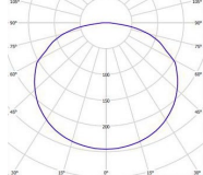
а) Косинусная (Д) - для светильников ЭСТ К-С-Д
