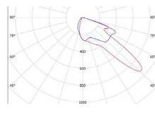
в) Глубокая (Г) - для светильников ЭСТ К-Х-Г
