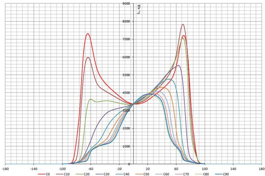
Рисунок 2. Декартовы координаты
