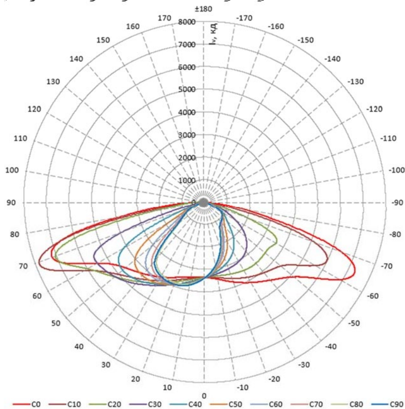
Рисунок 1. Полярные координаты
